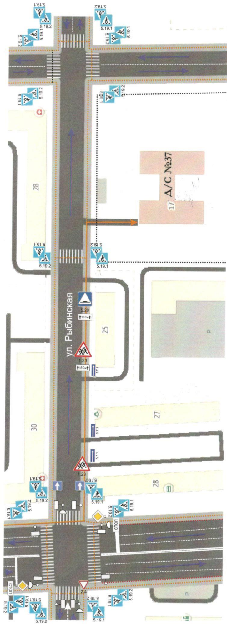
1.2. План-схема организации дорожного движения в непосредственной близости от МДОУ Детского сада №37 с размещением соответствующих технических средств, маршруты движения обучающихся и расположение парковочных мест
